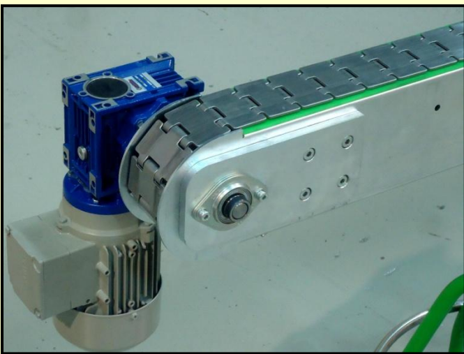
Aplicación limitada en anchura con cadena de 63 mm
