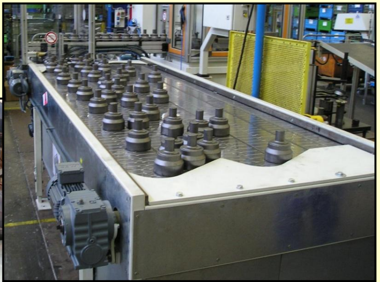
Líneas de avance opuesto para pulmón de piezas cilíndricas
