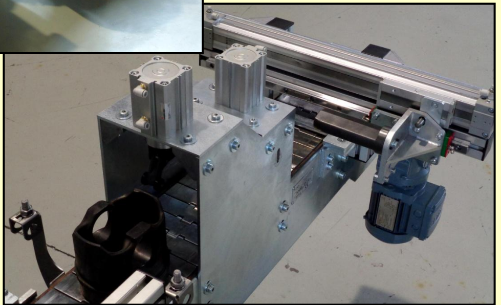
Dosificado de piezas a puesto de descarga por robot
