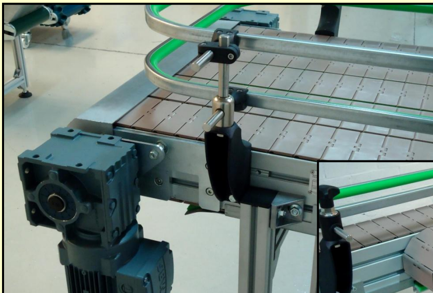
Pulmón de acumulación en salida de línea
