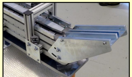
Rampa de entrada de piezas con 2 hileras
