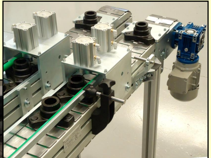
Dosificado de piezas a puesto de descarga por robot
