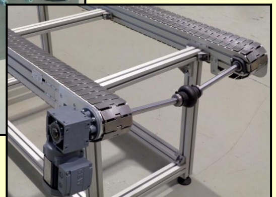
Doble hilera con motor común y eje motriz recto o inclinado
