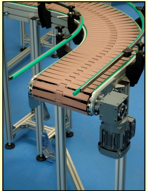
Curva de 90º con Ancho de 305 mm
