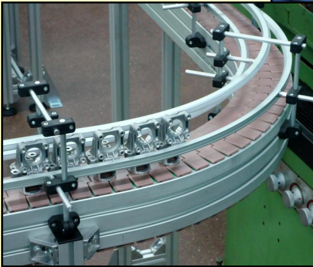
Guiado de pieza anti-giro en acumulación
