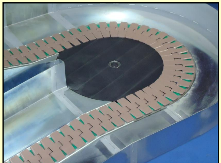
Cadena de giro reducido (R200) con curva de 180º mediante plato
