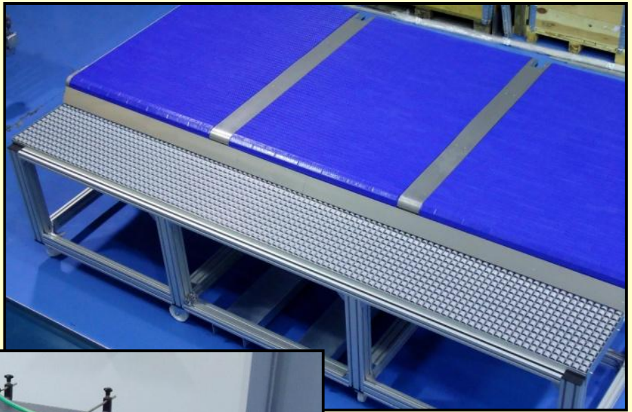
3 Hileras de Banda modular con carenado completo y mesa de roldanas
