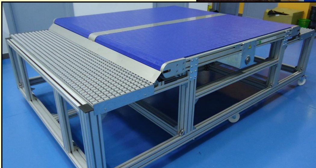
2 Hileras de Banda modular con mesa de roldanas y motorización central
