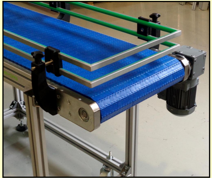
Mesa de salida en acumulación
