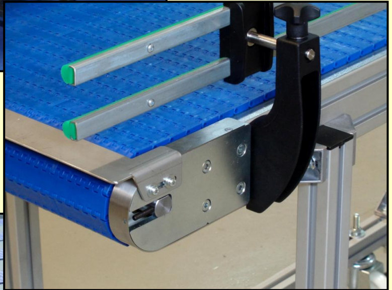
Chapa de paso de piezas en Acero Inoxidable
