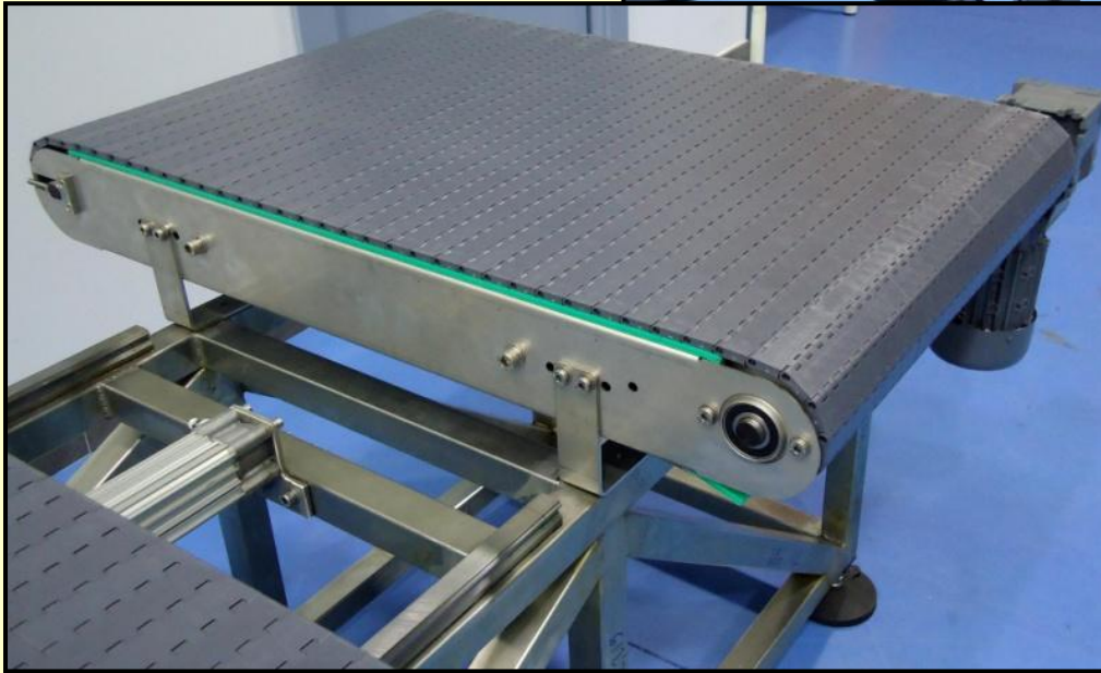
Banda modular con chasis de Acero Inoxidable
