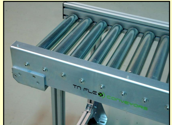
Rodillos Ø60 motorizados por cadena con paso de 80 mm
