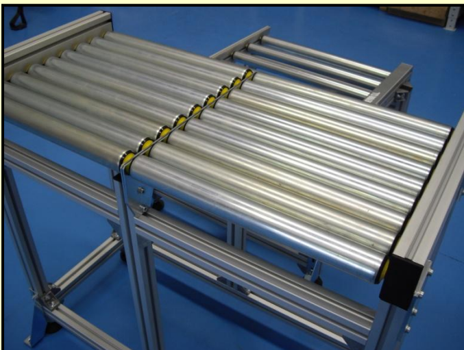
Rodillos Ø50 con paso de 60 mm
