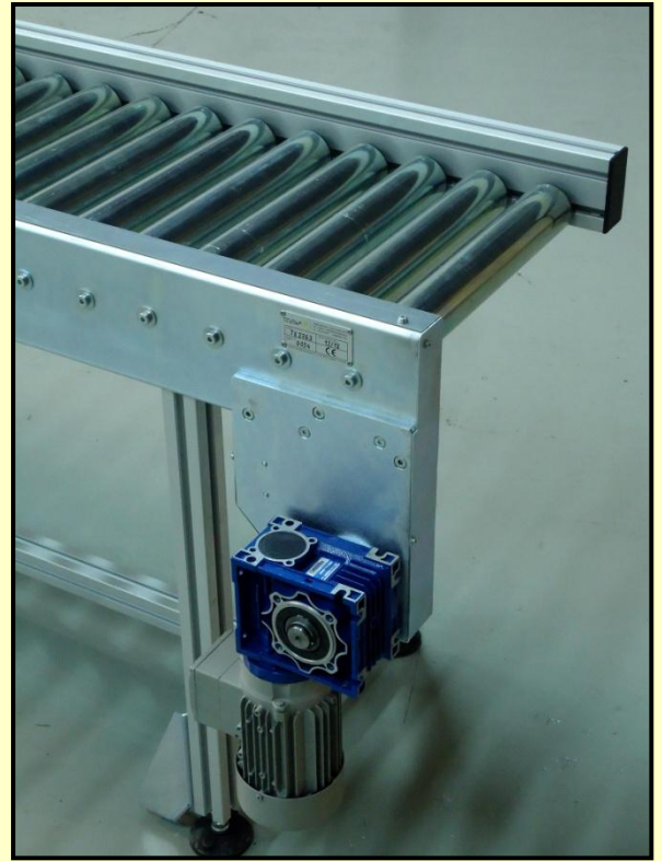
Rodillos Ø60 motorizados por cadena con paso de 80 mm
