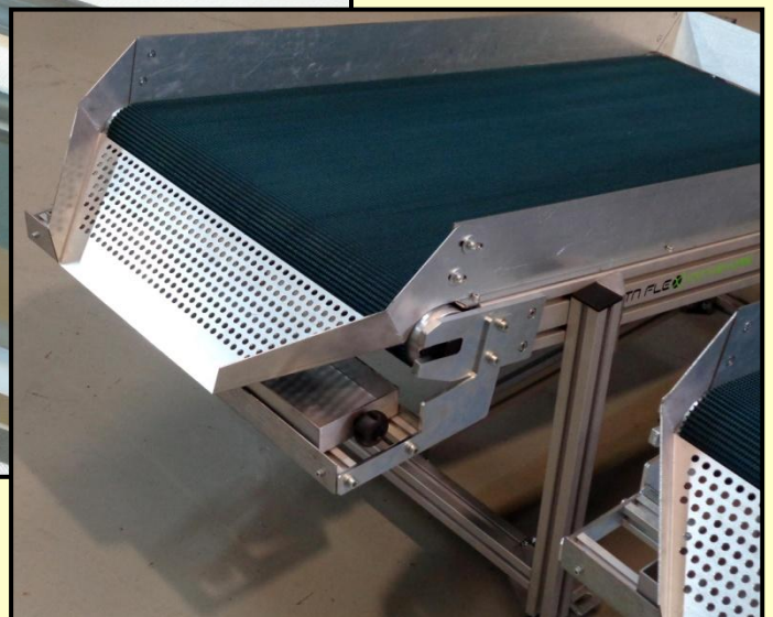
Pico de descarga perforado y cajón de recogida de granalla
