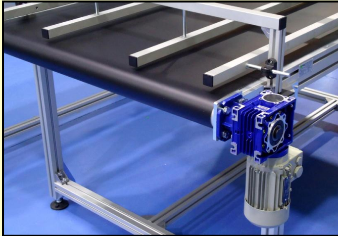
Separación en 4 vías mediante guiado superior
