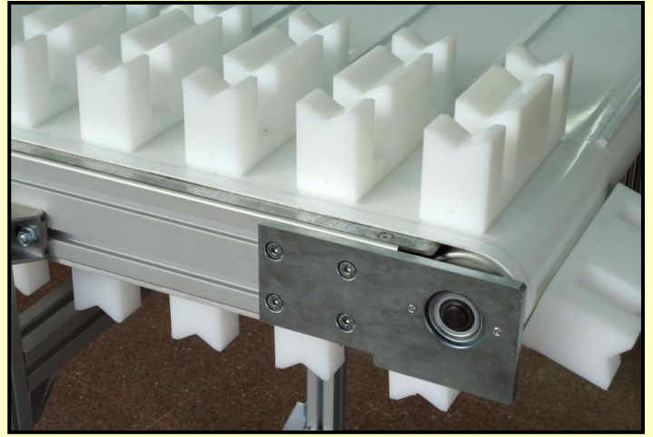
Separación en 4 vías mediante guiado superior
